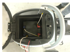
步骤3: 放入电池缓冲件并将 电池连接线牵引至缓冲件上方
