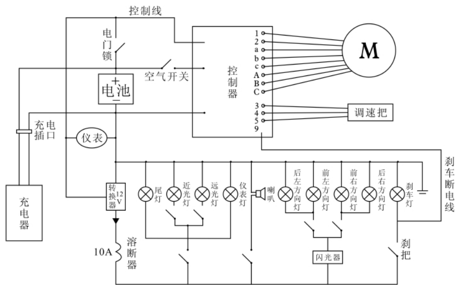
整车线路示意图
