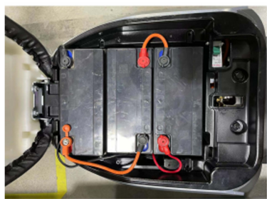
步骤 3: 将电池放入舱内，正确 把电源线进行连接
