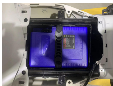
步骤2: 将锂电池合理摆放入电池盒体内。
