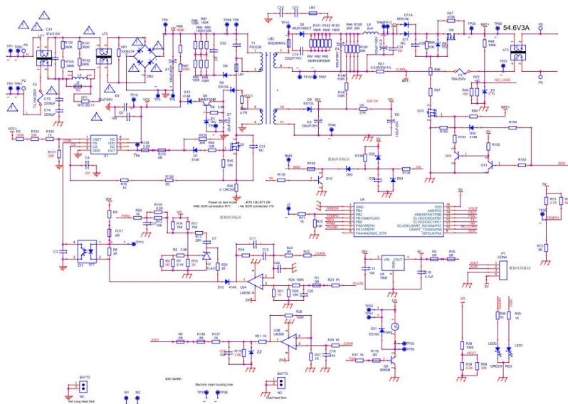
电气原理图
