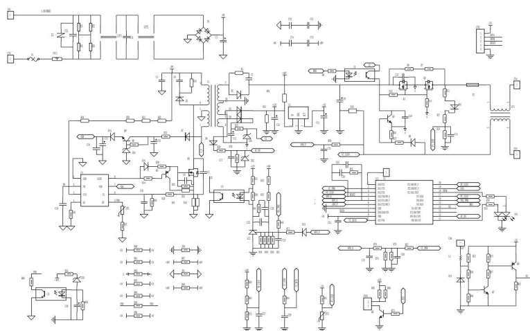
电气原理图
