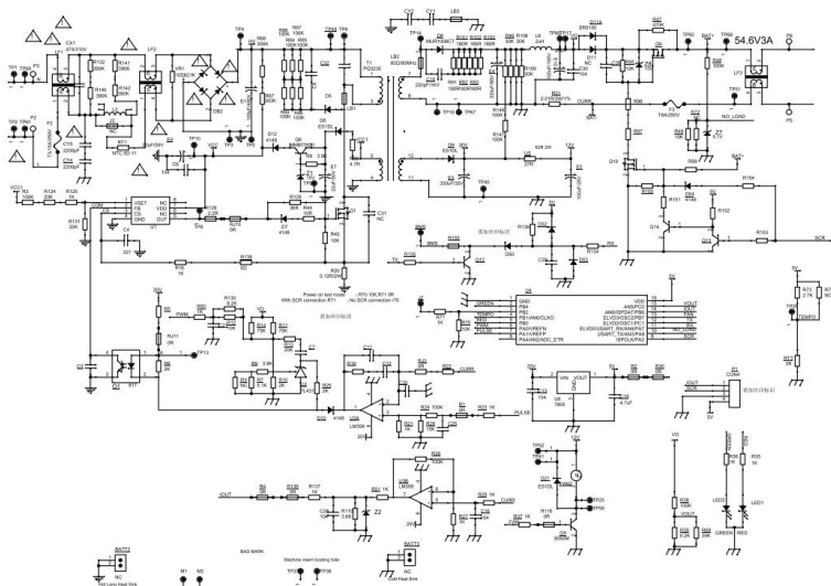
电气原理图
