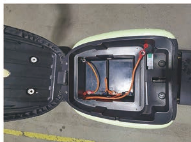
步骤 2: 使用电池连接线将 电池正确连接在一起
