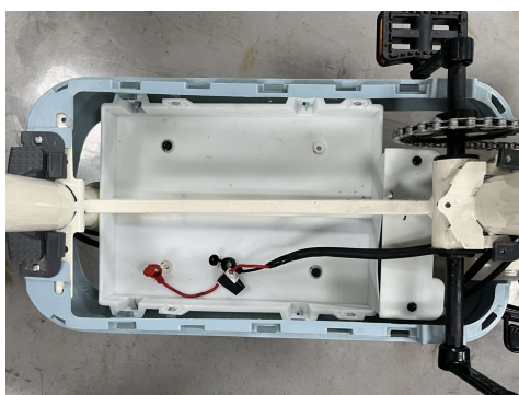
第三步：将电池盒安装到脚踏板内，并将充电器输出插头与主电缆连接
