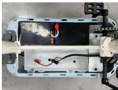
第四步：放入第一、二块电池并将电池连接线固定安装
