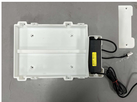
第一步：将车载充电器放入充电器卡槽内
