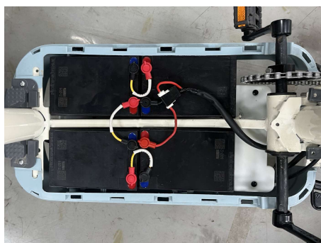
第五步：放入第三、四块电池并将电池连接线固定安装
