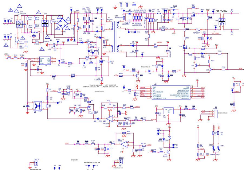
电气原理图
