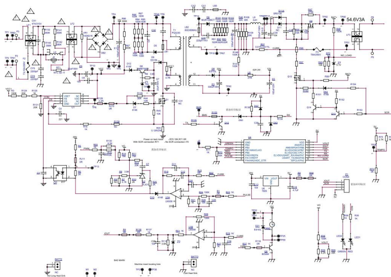
电气原理图
