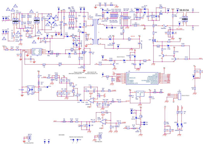
电气原理图
