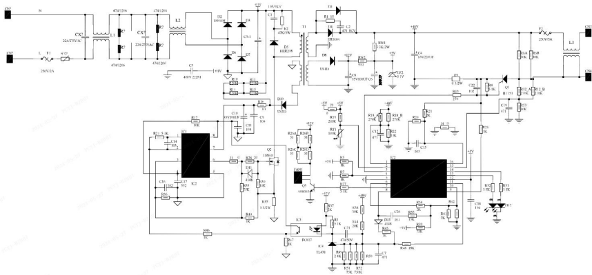
电气原理图
