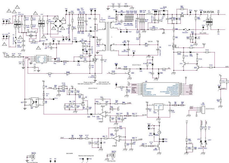
电气原理图
