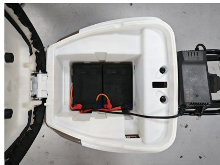
第四步：放入第三、四块电池 并将电池连接线安装
