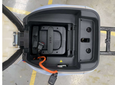
第二步：放入电池
