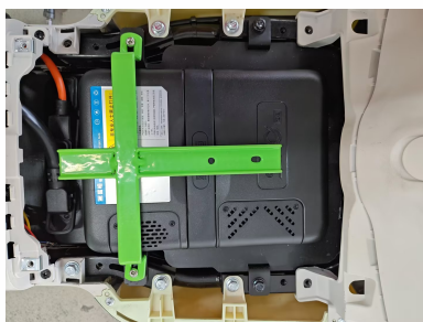
步骤3：把电池线插入电池 接通电源 用防篡改螺丝紧固 电池压条和固定电池
