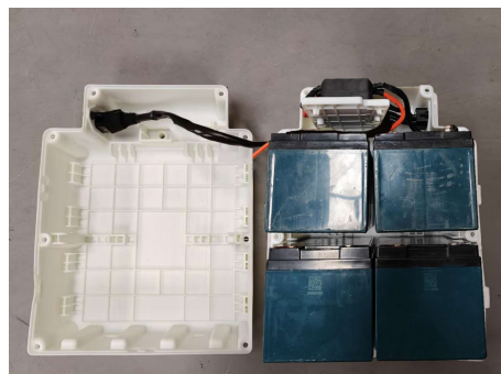
第二步：装入电池并正确连接电源线
